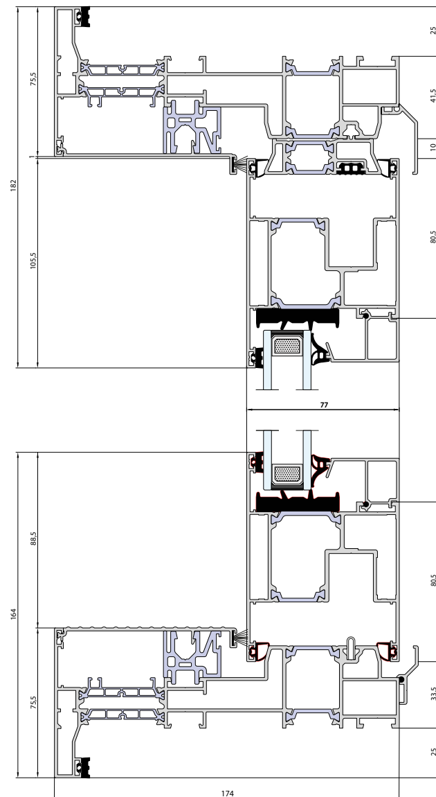
schuifdeur
